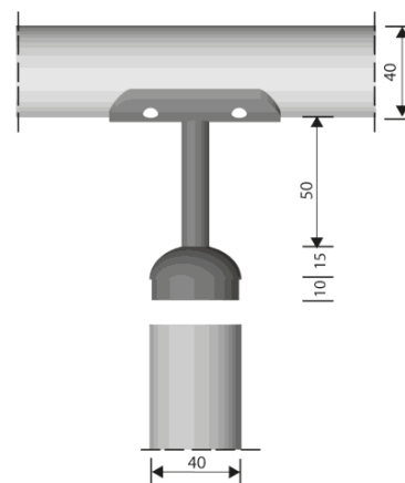
Yläpään kiinnike Pystypilarin ja käsijohteen välille. Suositeltava tukiväli on 1,2 m.
