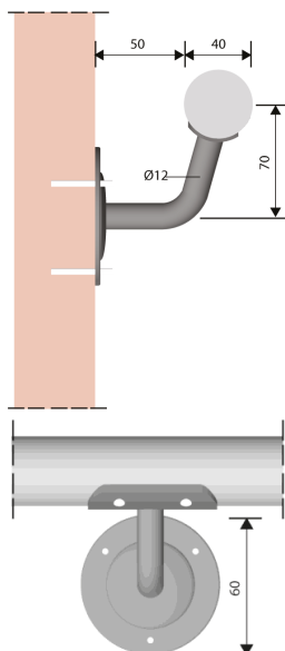
Ruuvikiinnitteinen seinäkannake Puuseiniin ja teräsrakenteisiin. Suositeltava asennusväli on 1,2 m
