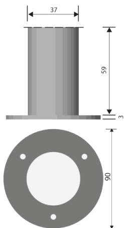
Pilarikiinnike Pystypilarin alapään kiinnike esim. lattiakiinnityksiin
