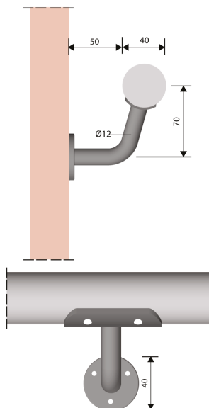
Seinäkannake ruuveilla Normaalia kapeampiin puu- tai teräsrakenteisiin. Suositeltava asennusväli on 1,2 m.
