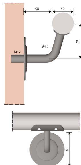
Seinäkannake M2 Tarkoitettu esim. betoniseiniin. Suositeltava asennusväli on 1,2 m.
