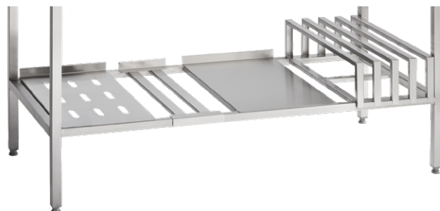
Kuvassa hyllyvaihtoehdot: reikälevyhylly, ritilähyllyillä, tasohylly sekä teline leikkuulautoille.
