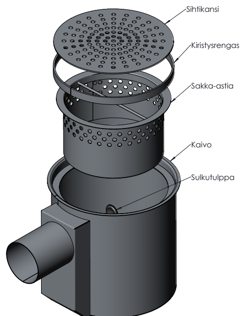
Kuvassa pönttökaivo 9081/1
