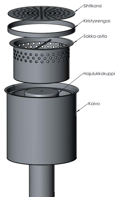
Kuvassa pönttökaivo 9083/1
