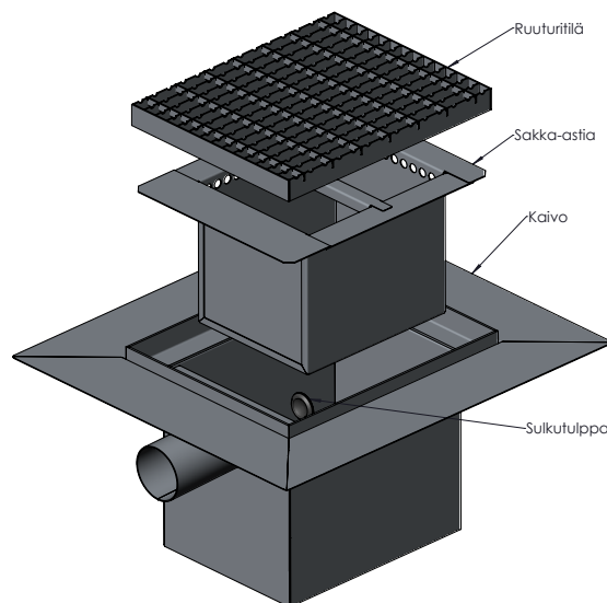
Kuvassa hiekanerotuskaivo 9070/1
