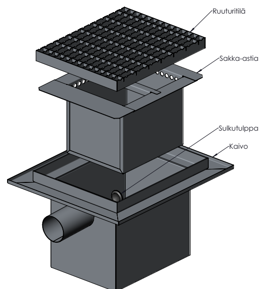
Kuvassa hiekanerotuskaivo 9070/4
