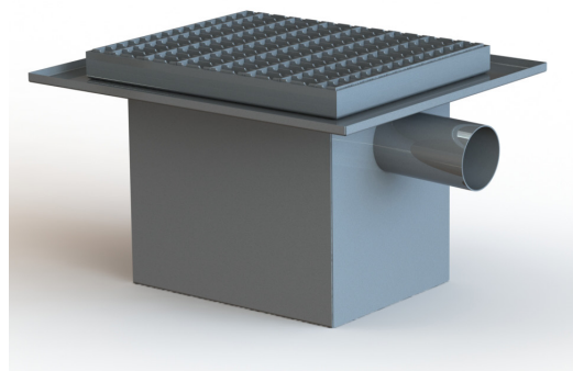
Kuvassa hiekanerotuskaivo 9070/4
