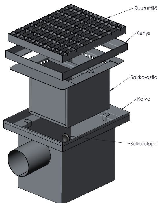
Kuvassa hiekanerotuskaivo 9071/1
