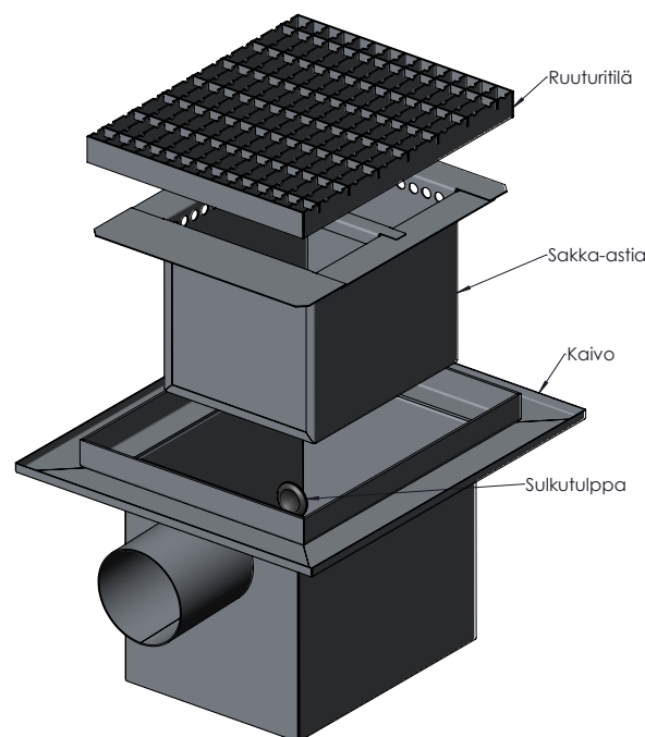
Kuvassa hiekanerotuskaivo 9071/3X
