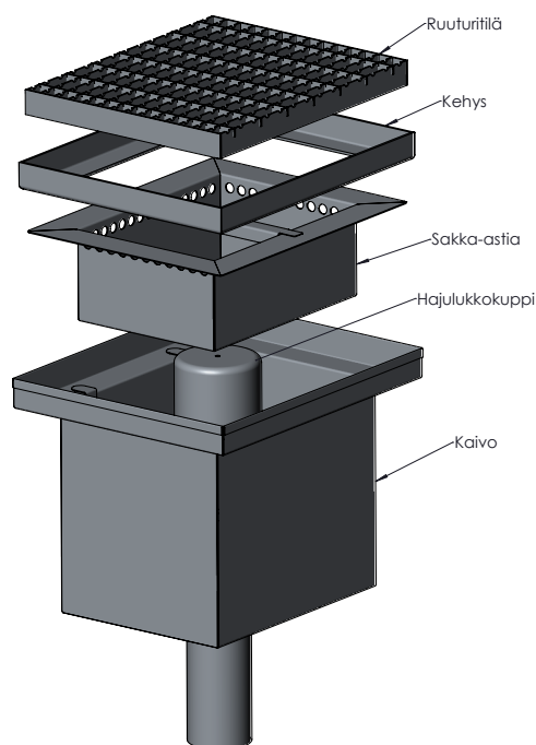
Kuvassa hiekanerotuskaivo 9072/1
