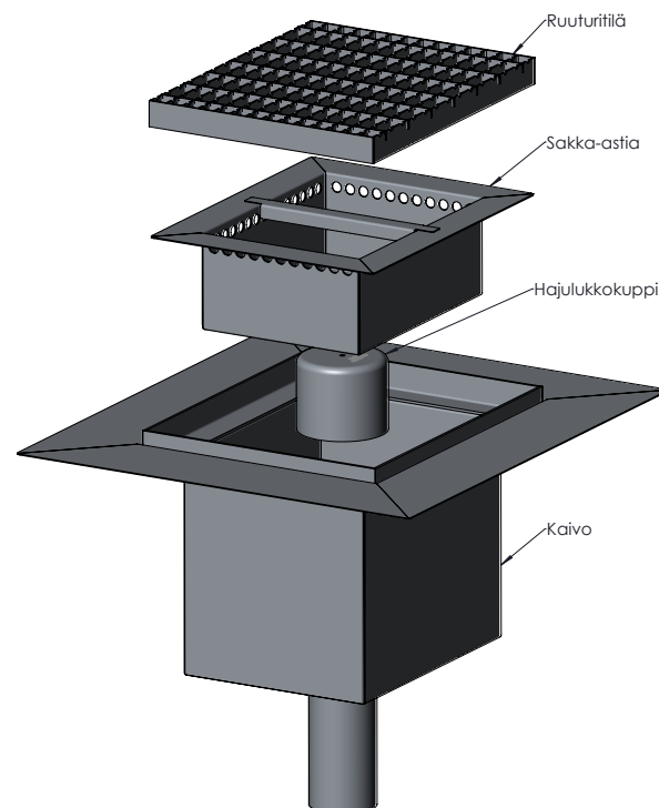
Kuvassa hiekanerotuskaivo 9072/3X
