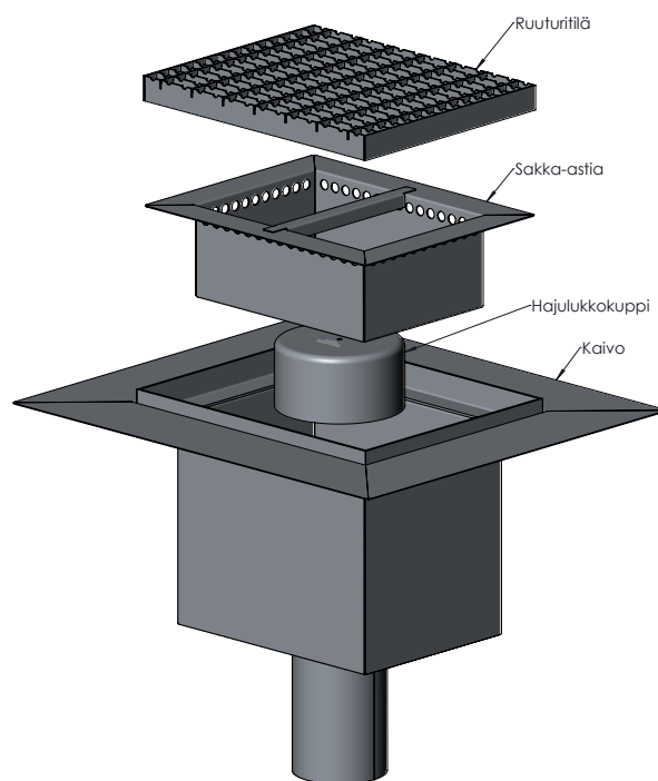
Kuvassa hiekanerotuskaivo 9073/3X
