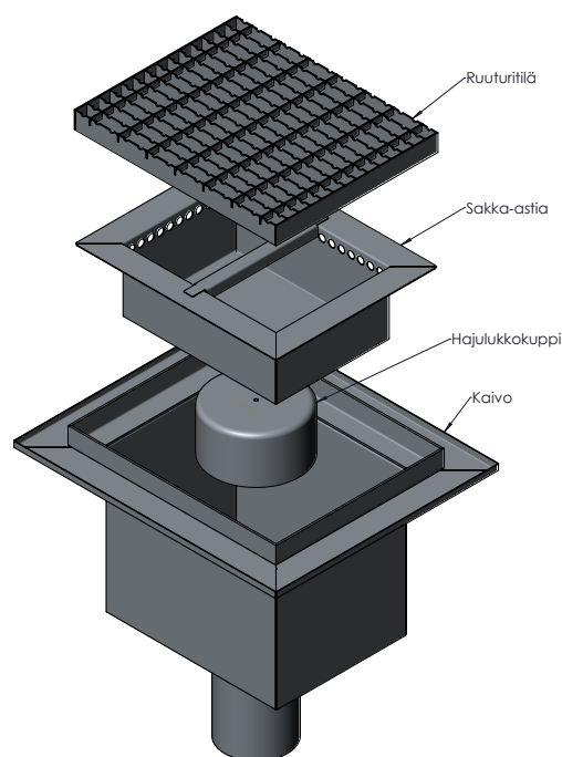
Kuvassa hiekanerotuskaivo 9073/4
