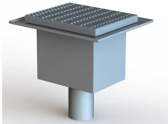
Kuvassa hiekanerotuskaivo 9073/4
