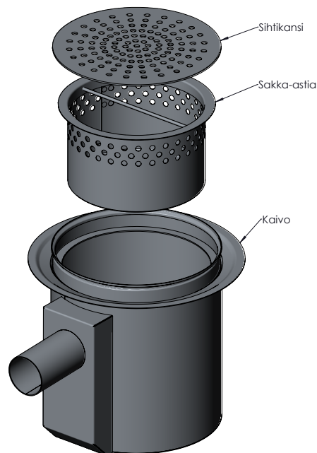
Kuvassa pönttökaivo 9080/4
