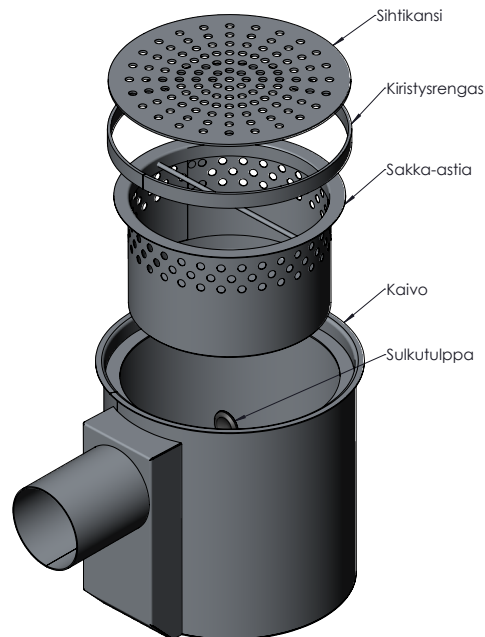
Kuvassa pönttökaivo 9081/1
