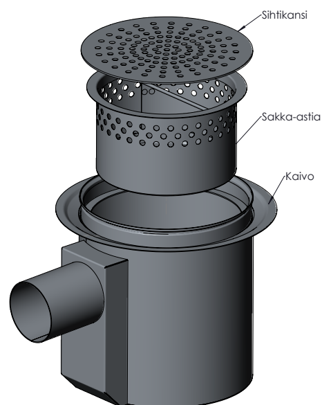
Kuvassa pönttökaivo 9081/4
