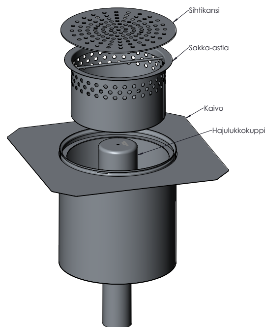
Kuvassa pönttökaivo 9082/3X
