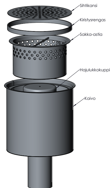
Kuvassa pönttökaivo 9083/1
