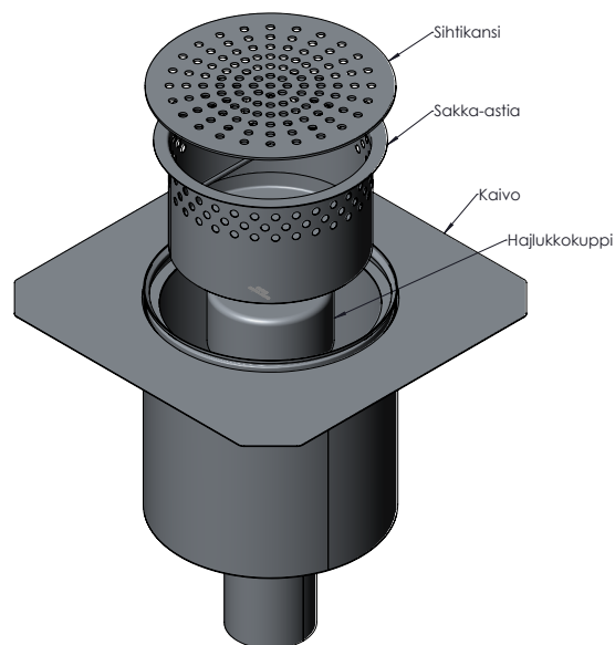
Kuvassa pönttökaivo 9083/3X
