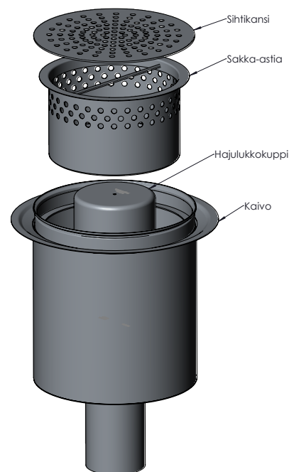
Kuvassa pönttökaivo 9083/4
