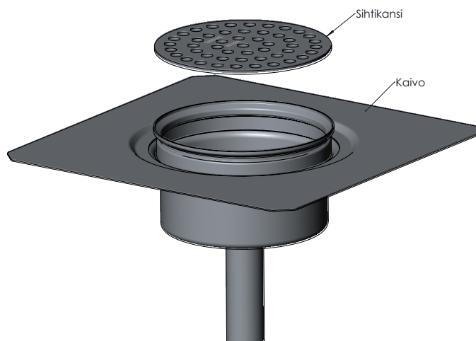
Kuvassa pystykuivakaivo 9053/3X
