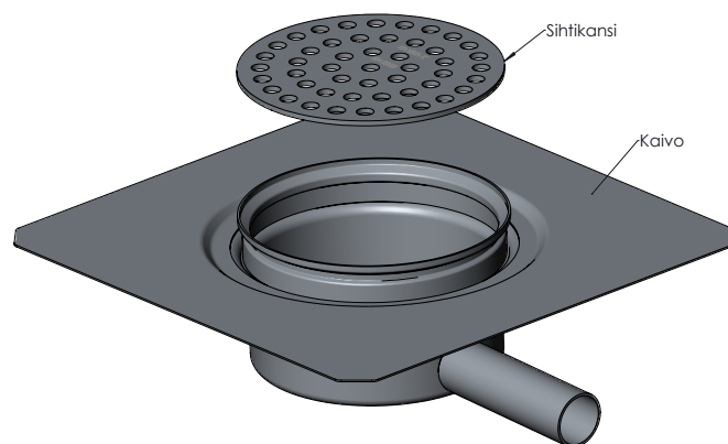
Kuvassa vaakakuivakaivo 9052/3X
