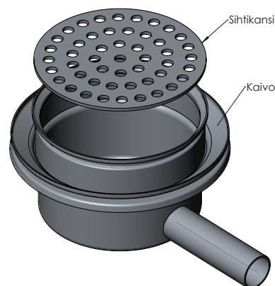
Kuvassa vaakakuivakaivo 9052/4
