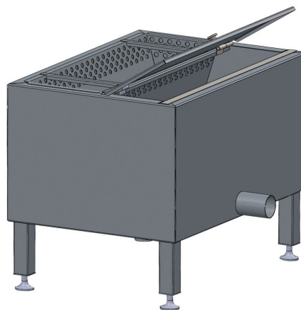
Kuvassa hiekanerotusallas 7077
