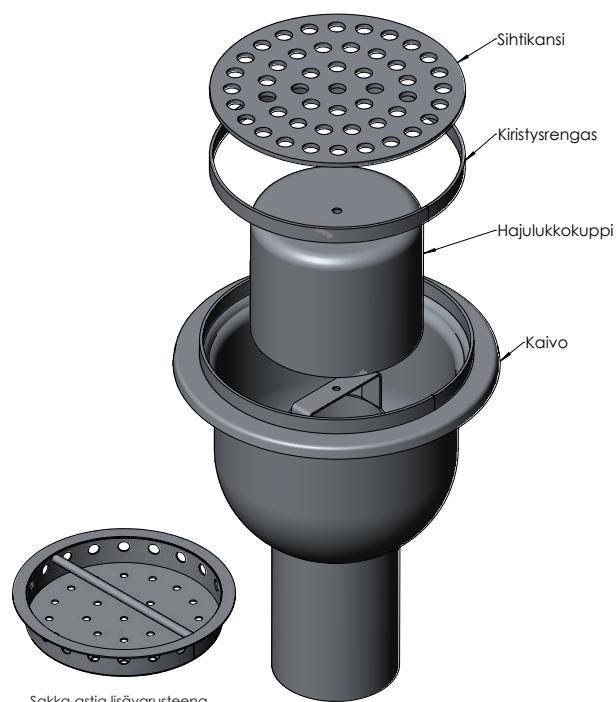
Kuvassa pystykaivo 9090/1
