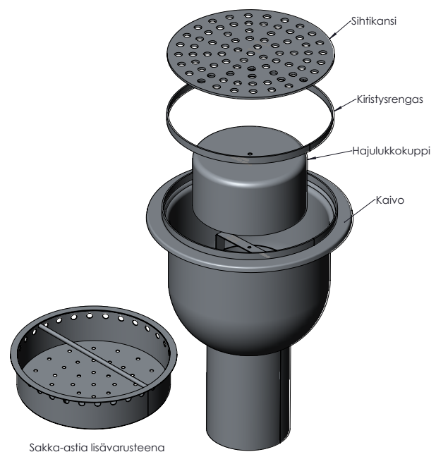
Kuvassa pystykaivo 9091/1
